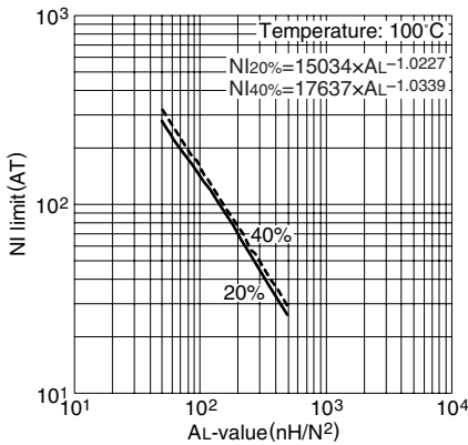
NI limit vs. AL 值(代表例) PC47ETD19 磁心(带空隙)
