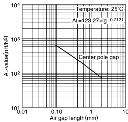
AL 值 vs. 气隙长度(代表例) PC47ETD29 磁心
