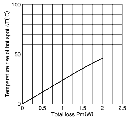
温度上升 vs. 总损耗特性(代表例) ETD29 磁心
