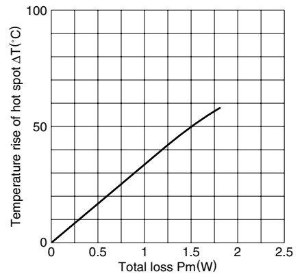
温度上升 vs. 总损耗特性(代表例) ETD19 磁心
