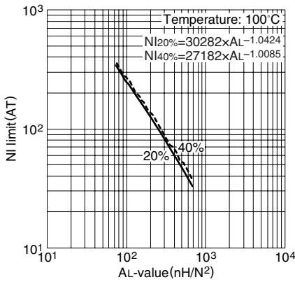
NI limit vs. AL 值(代表例) PC47ETD29 磁心(带空隙)
