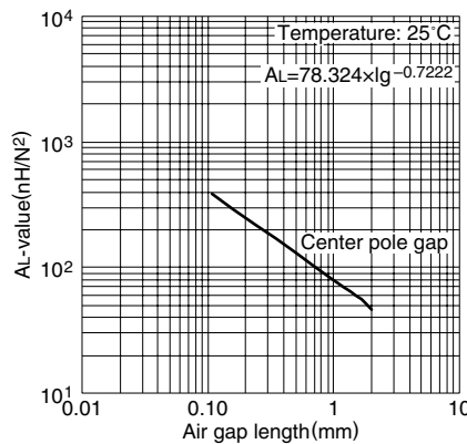
AL 值 vs. 气隙长度(代表例) PC47ETD19 磁心
