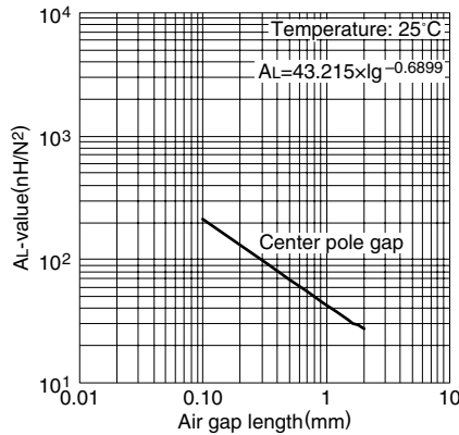
AL 值 vs. 气隙长度(代表例) PC47EE16 磁心
