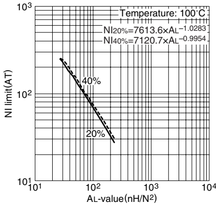
NI limit vs. AL 值(代表例) PC47EE16 磁心(带空隙)
